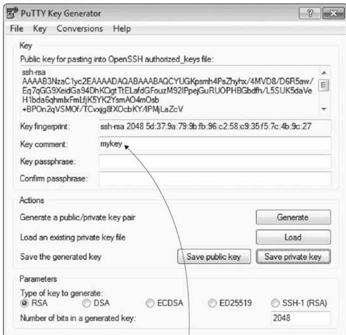
Rysunek 1.27. Narzędzie PuTTYgen pozwala skonwertować pobrany plik .pem na format wymagany przez program PuTTY, czyli .ppk
