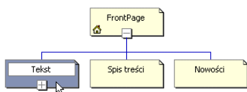
Rysunek 3.22. Poddrzewo można przesunąć nawet gdy jest ono zwinięte (strona ze zwiniętym poddrzewem posiada symbol +) — wystarczy kliknąć i przesunąć widoczną stronę
